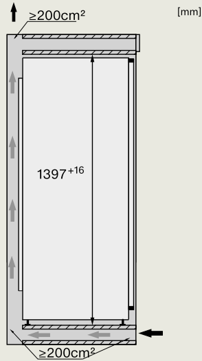
K 7437 D, K 7438 D, K 7447 C, K 7448C
